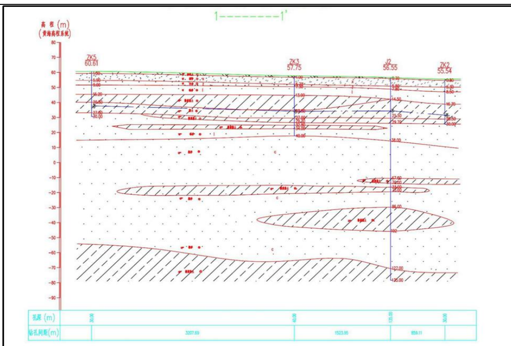
图 12 I—I'水文地质剖面图
