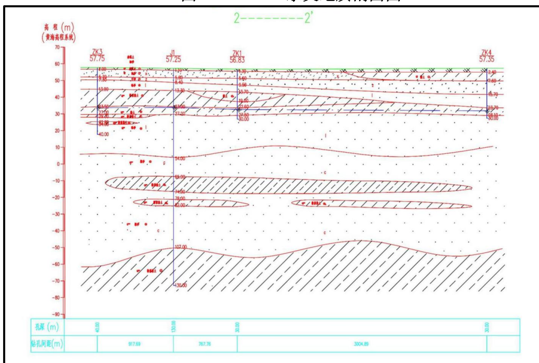
图 13 2—2'水文地质剖面图
