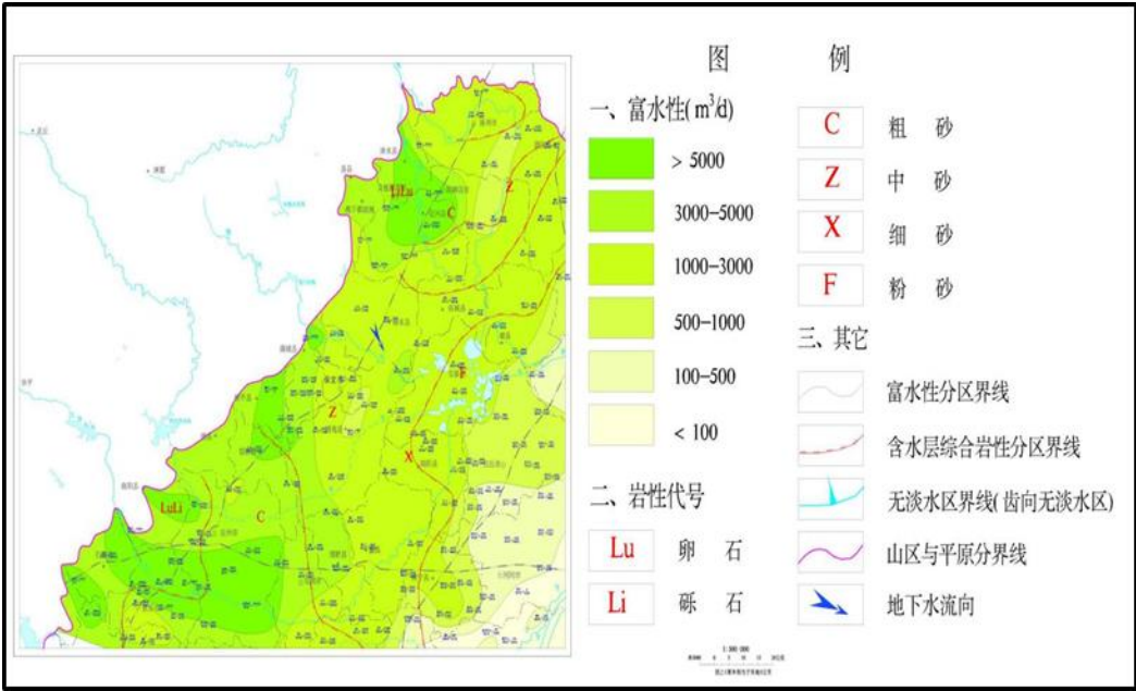
图 11 区域水文地质图
