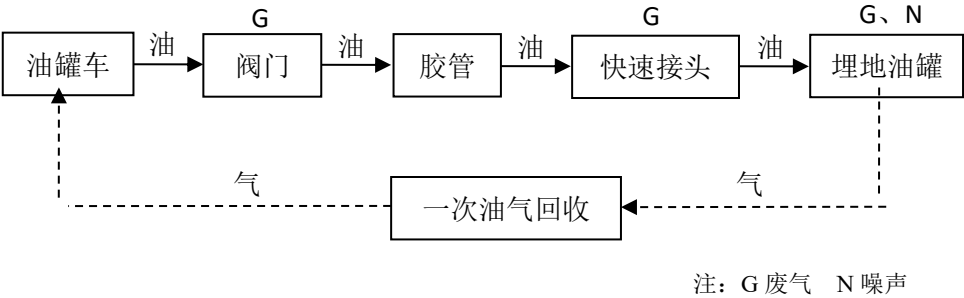
图 3 卸油工艺流程及排污节点
