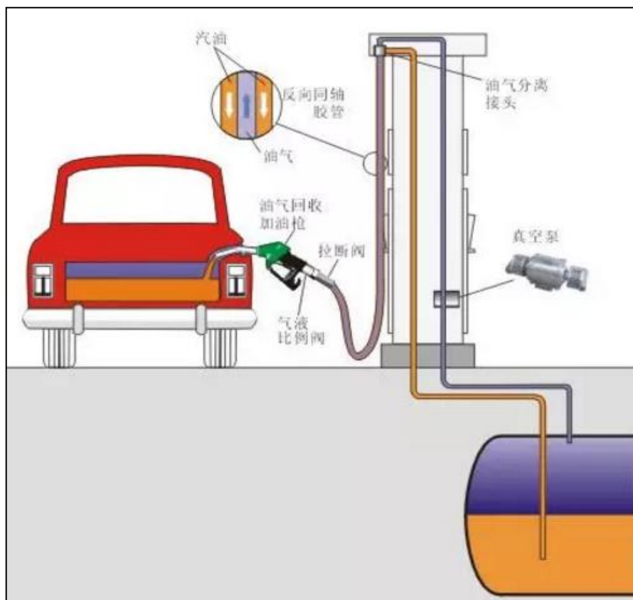
图 6 分散式二次油气回收系统示意图
