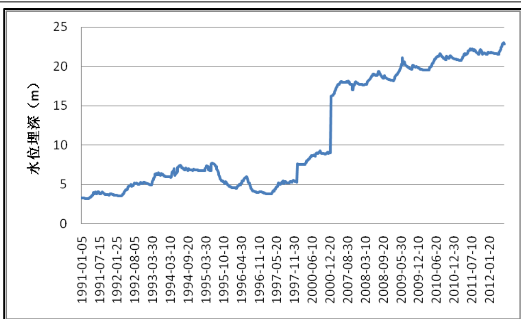
图 14 西城乡支白土村北地下水监测点水位动态曲线
