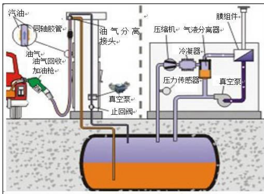
图 8 油气排放装置示意图
