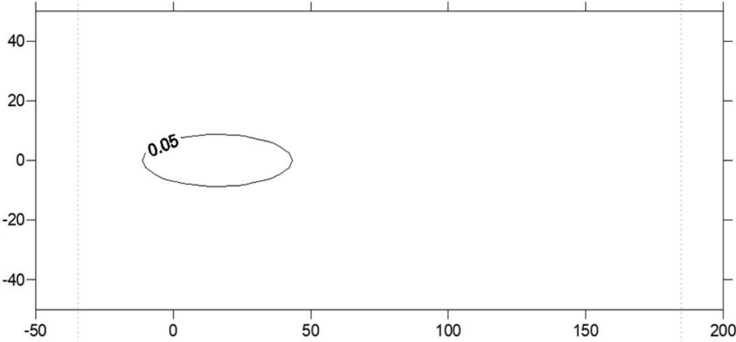
图 15 含水层中污染晕影响范围图
