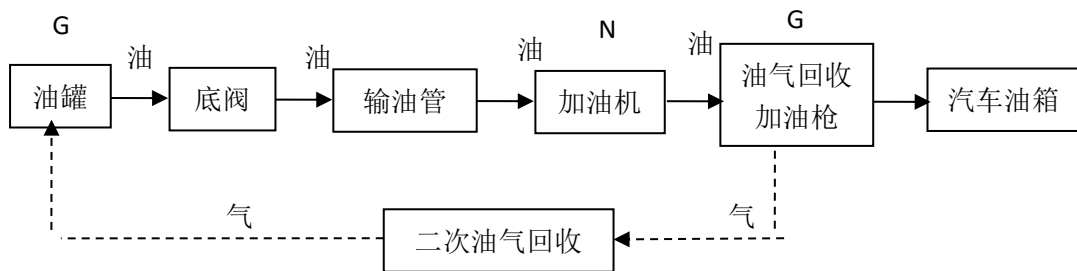
图 2 加油工艺流程及排污节点
