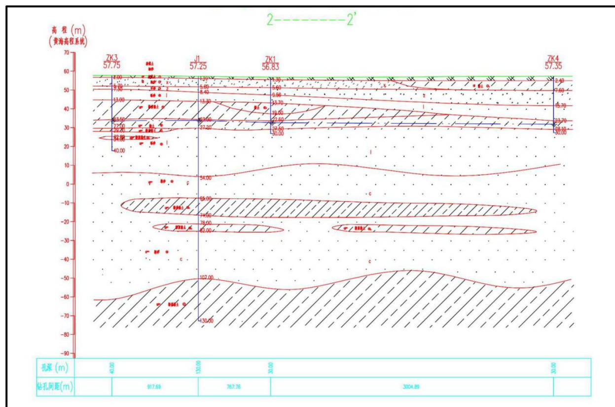
图 11 2—2'水文地质剖面图
