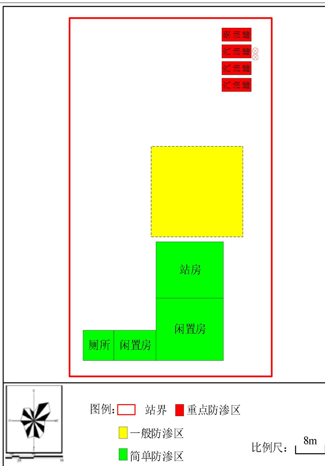
图 14 项目分区防渗布置图
