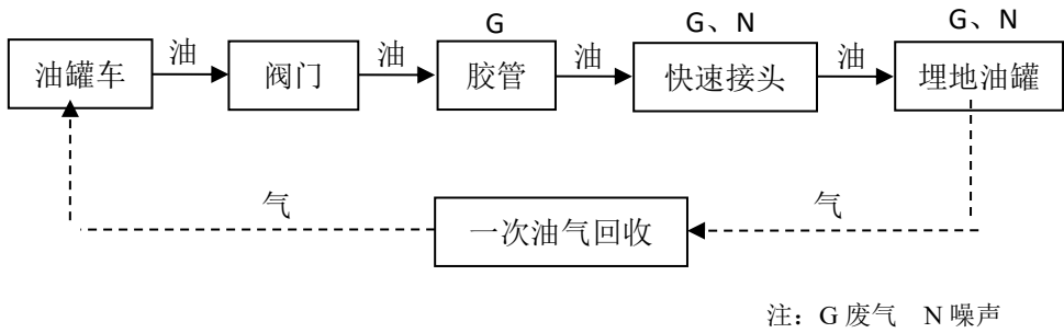
图 1 卸油工艺流程及排污节点
