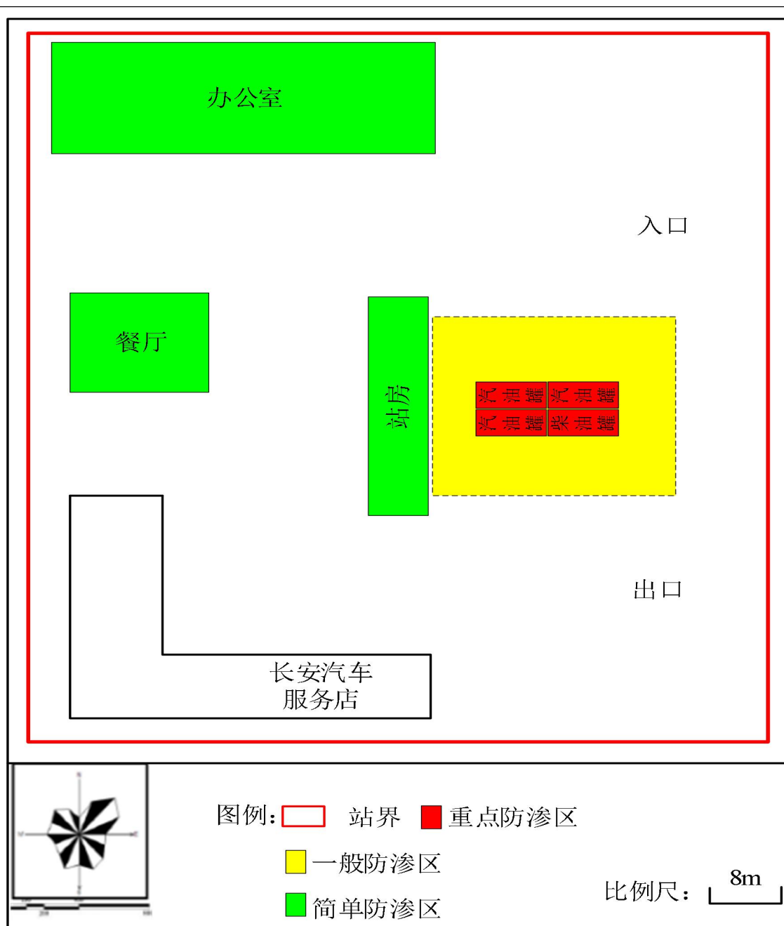
图 14 项目分区防渗布置图
