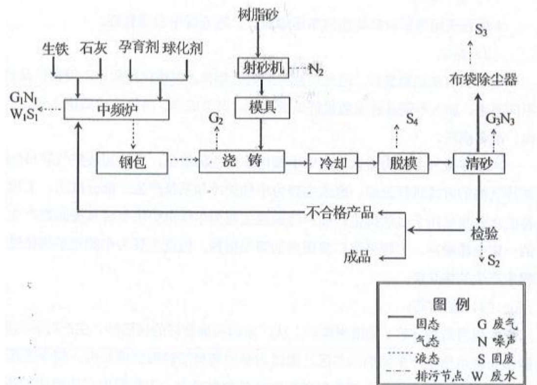
图2 现有工程生产工艺流程图
