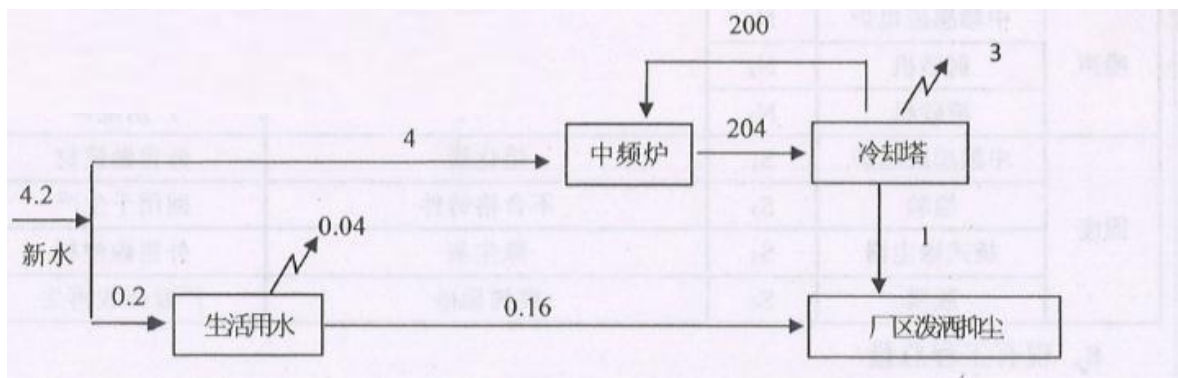
图 1 现有工程给排水平衡图
