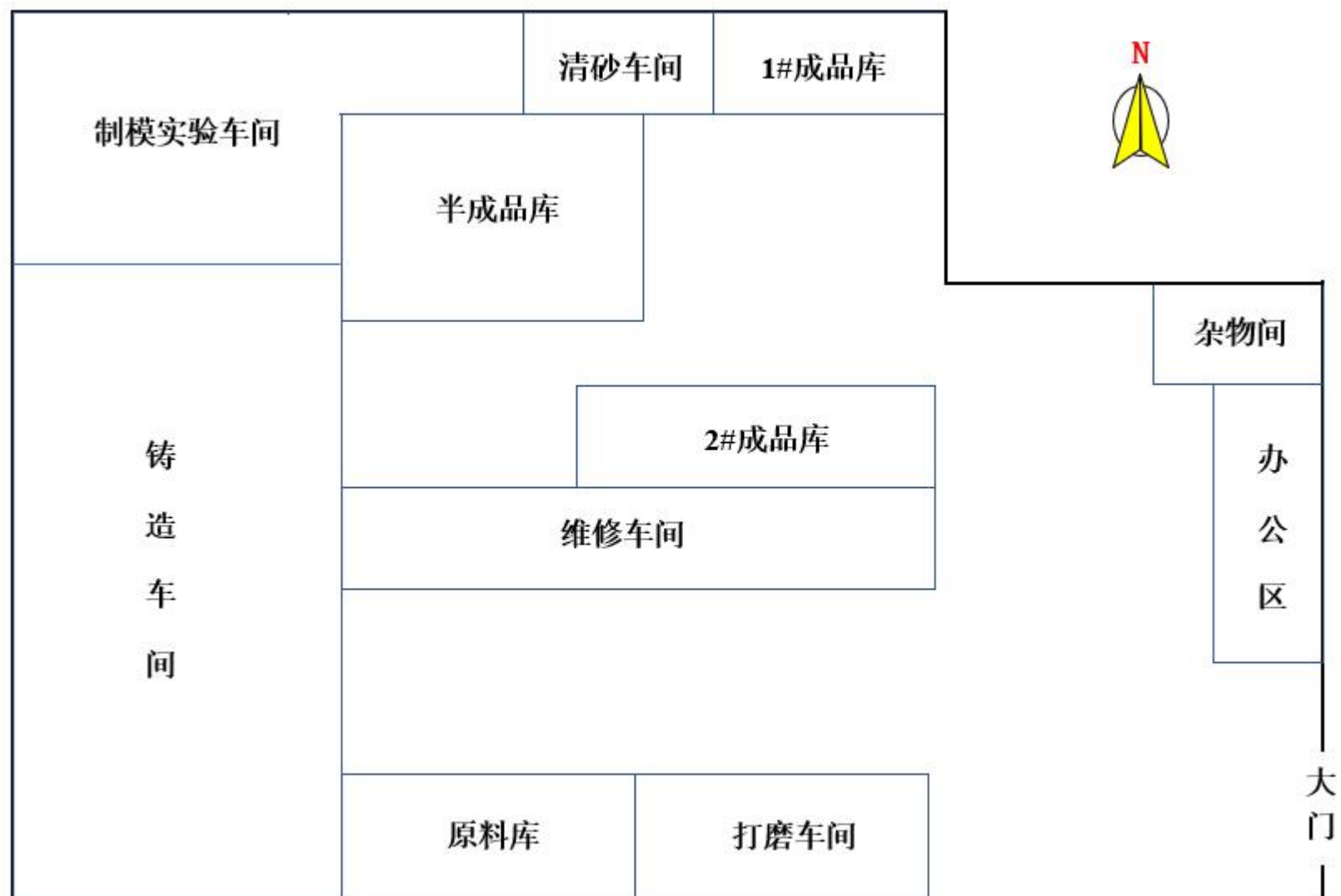
附图 3 技改后本项目厂区平面布置图
