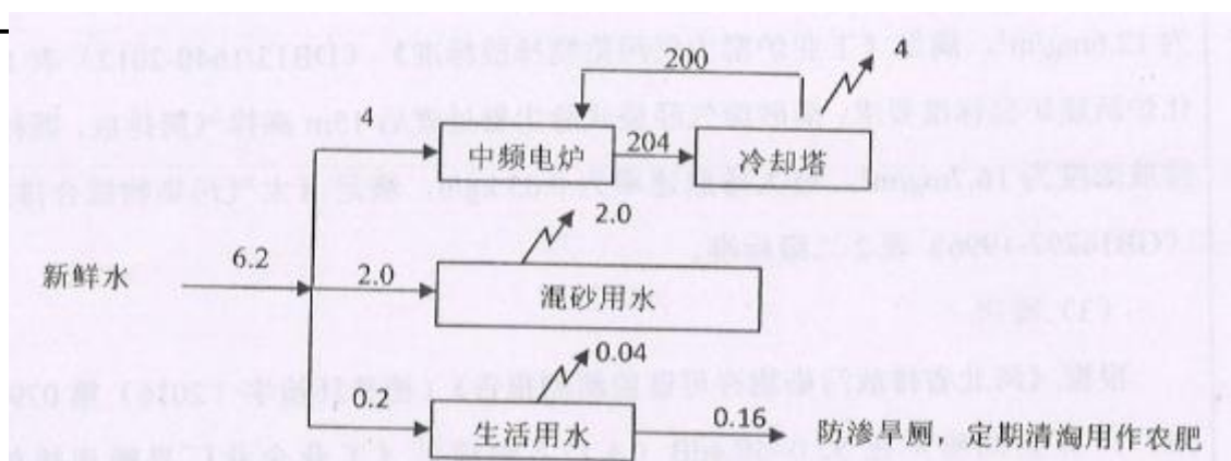
图3 技改后全厂给排水平衡图
