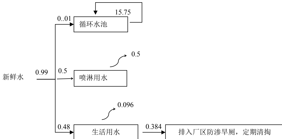
图1 本项目水平衡图（单位：m³/d）
