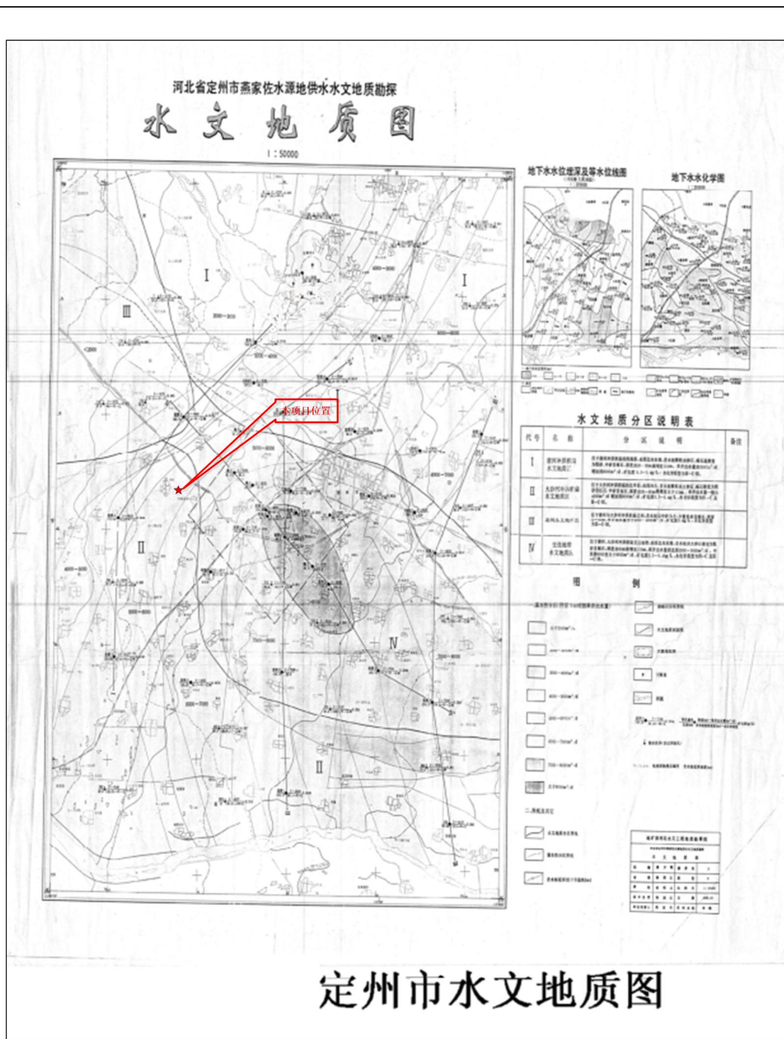
5 定州市水文地质图
