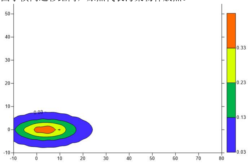
图 8 石油类污染晕运移 30 天影响范围图
