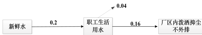
图 1 项目用水平衡图 单位 m 3 /d
