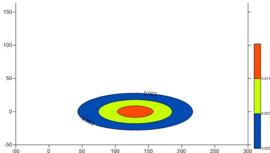
图 10 石油类污染晕运移 1000 天影响范围图
