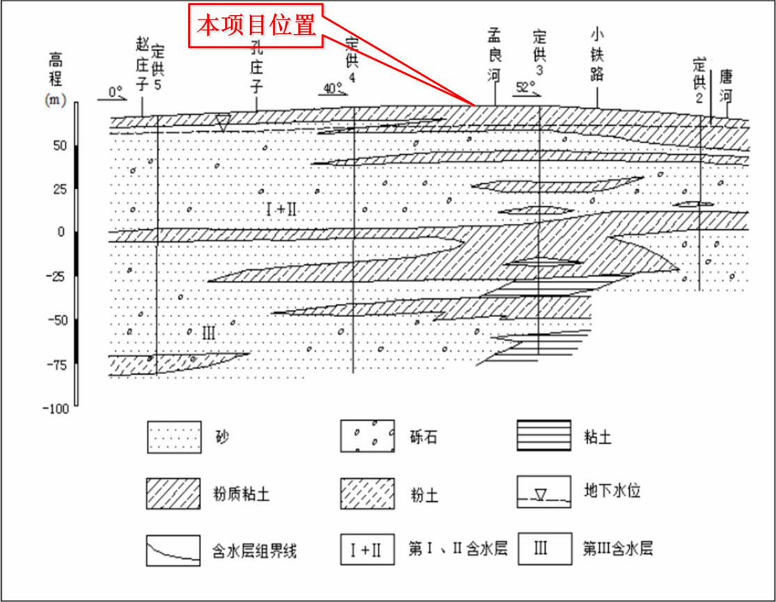
图 4 研究区水文地质剖面图
