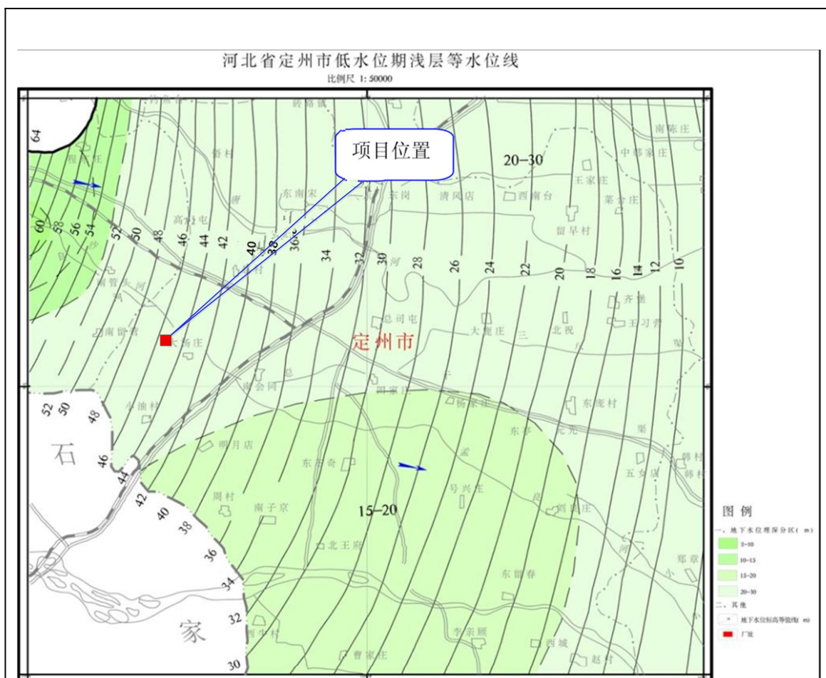
图 6 定州市低水位期浅层等水位线图
