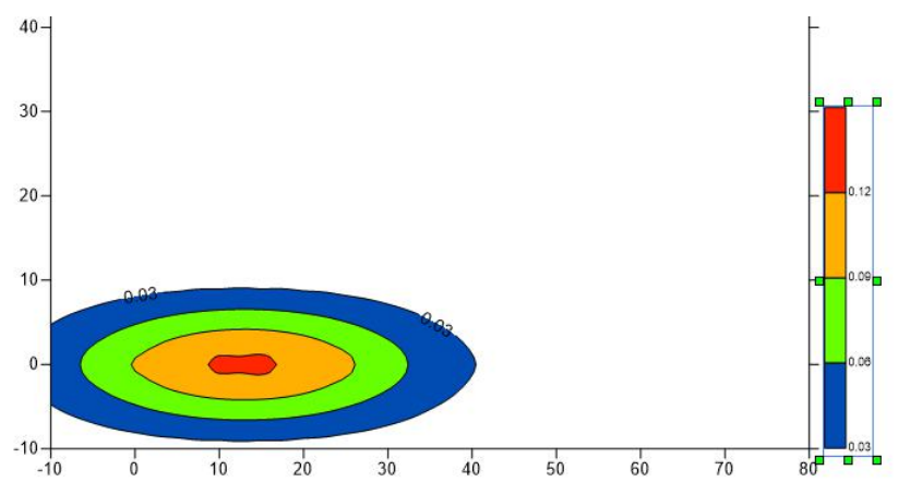
图 9 石油类污染晕运移 100 天影响范围图
