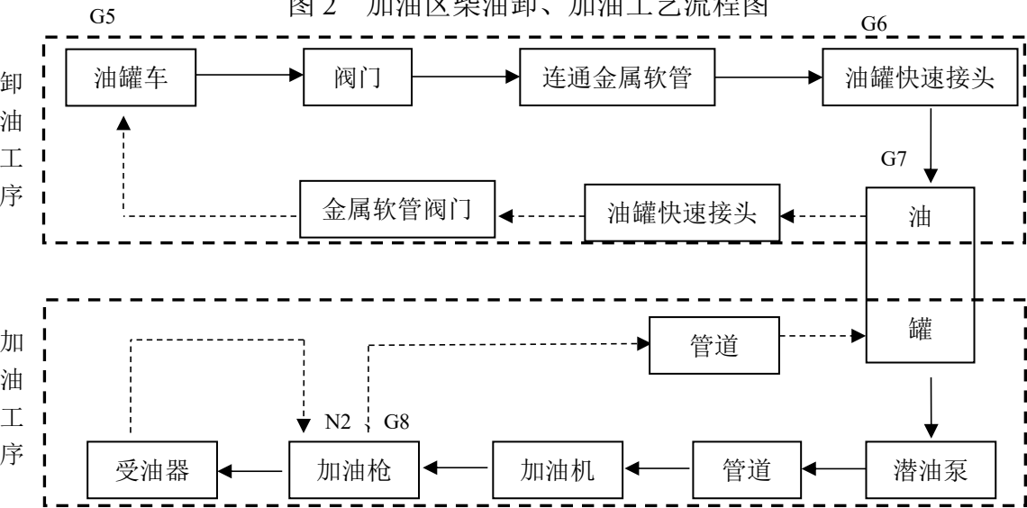
图 2 加油区柴油卸、加油工艺流程图
