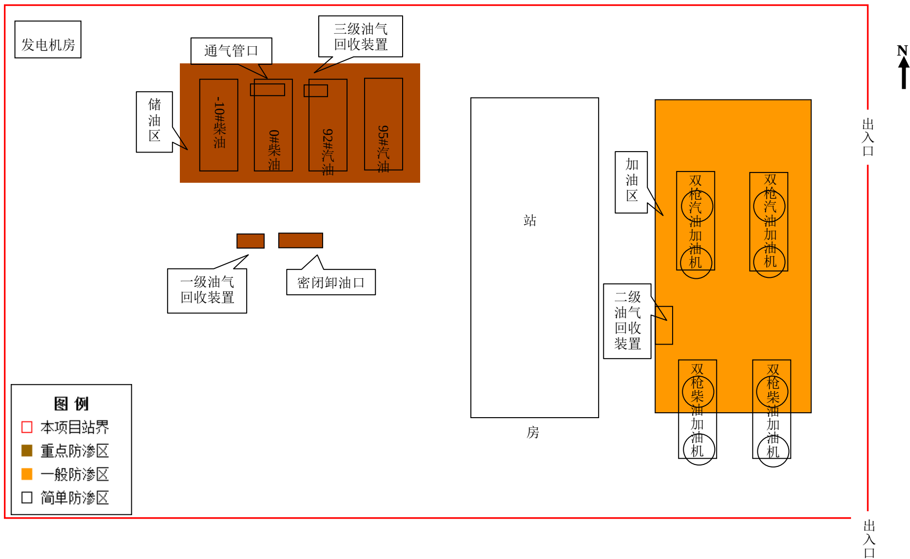
附图 3 建设项目总平面布置及防渗图
