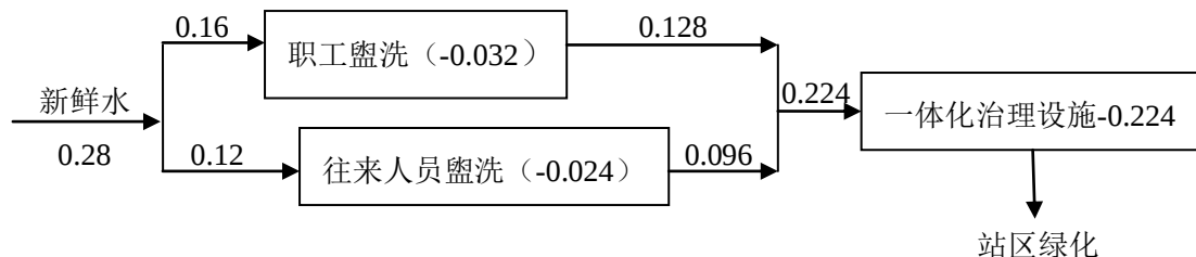
图 1 建设项目水量平衡图
