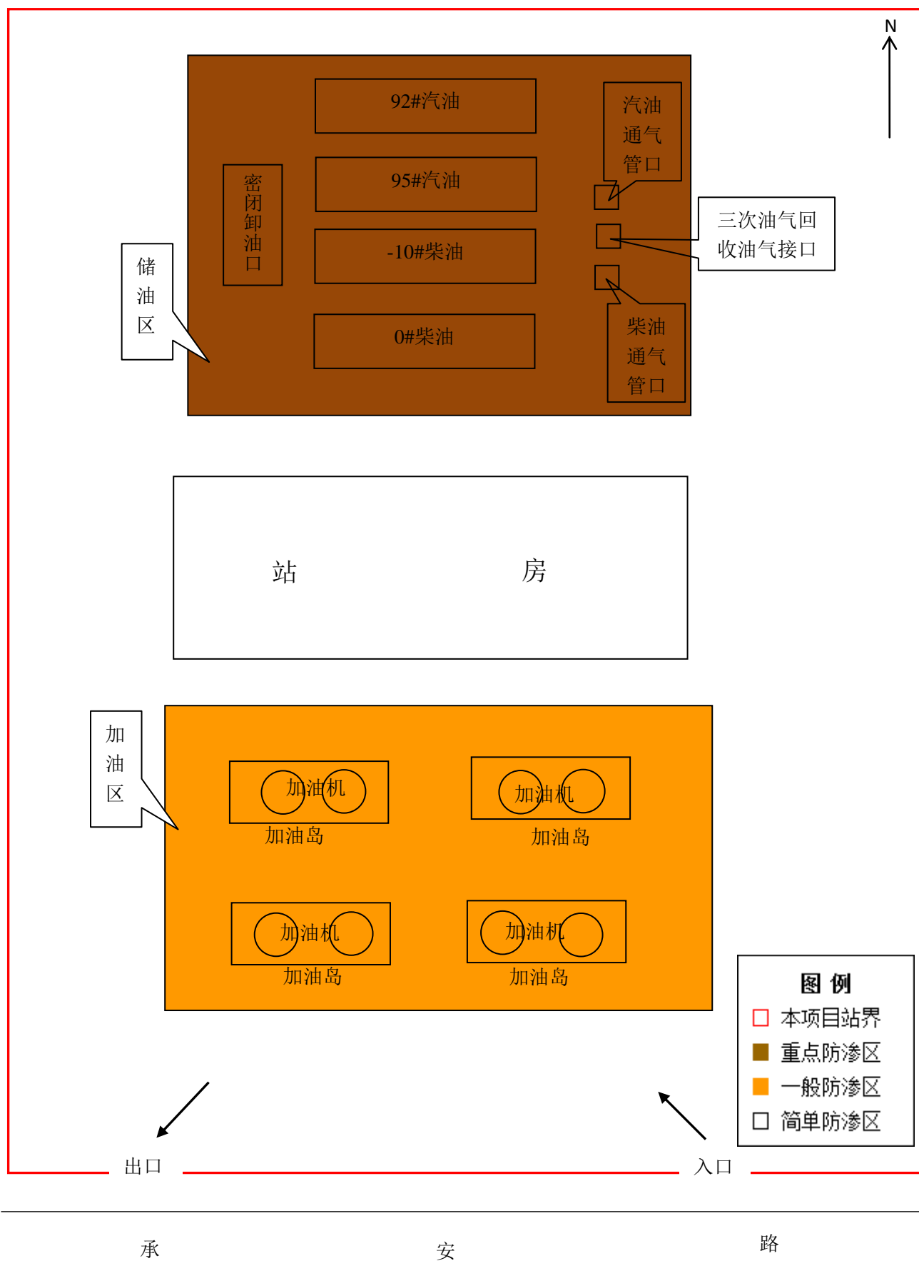
附图3 建设项目站区总平面布置图及防渗图
