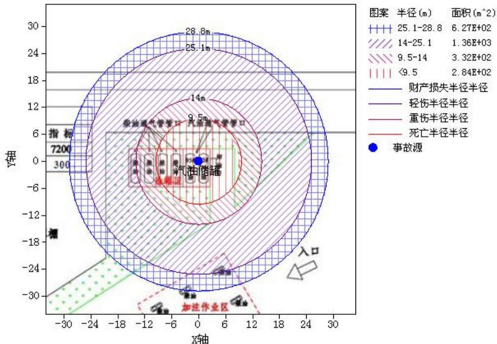
图 6 加油站汽油爆炸伤害范围图
