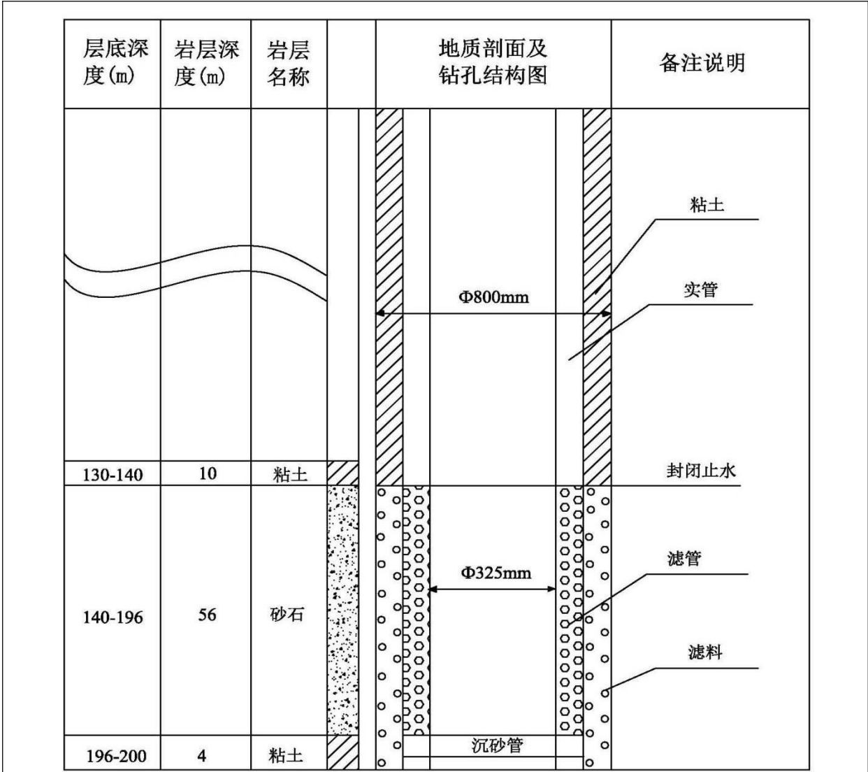
图 4-4 水井柱状图
