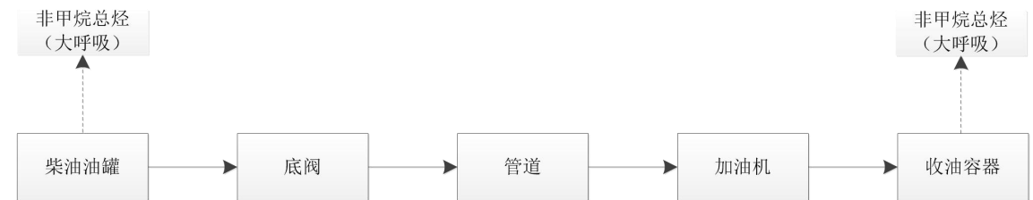
图 2 柴油加油工艺流程及产污节点图
