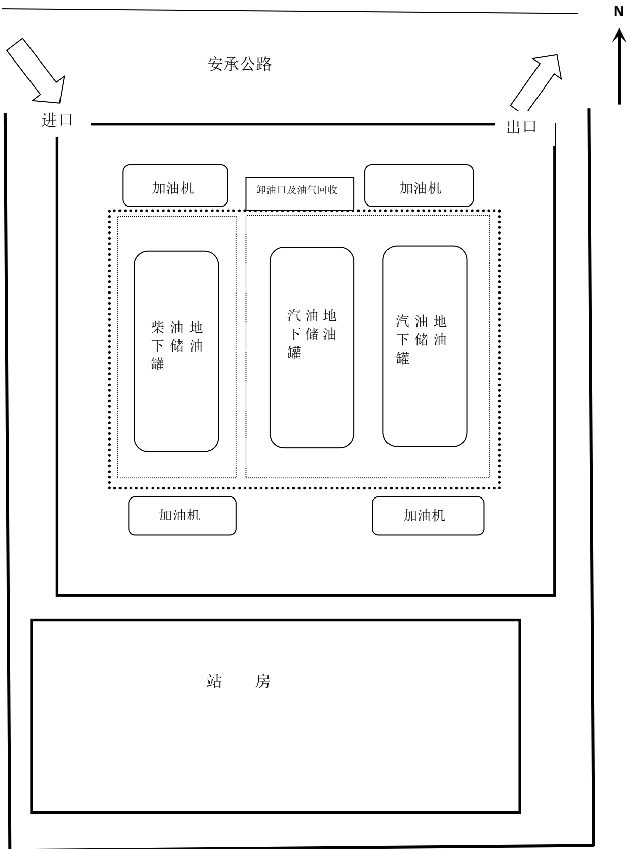
附图3 建设项目厂区总平面布置图
