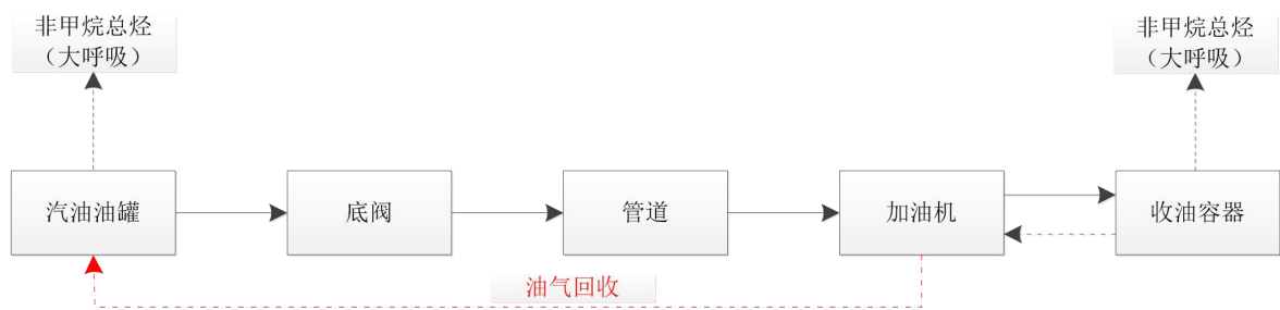
图4 汽油加油工艺流程及产污节点图
