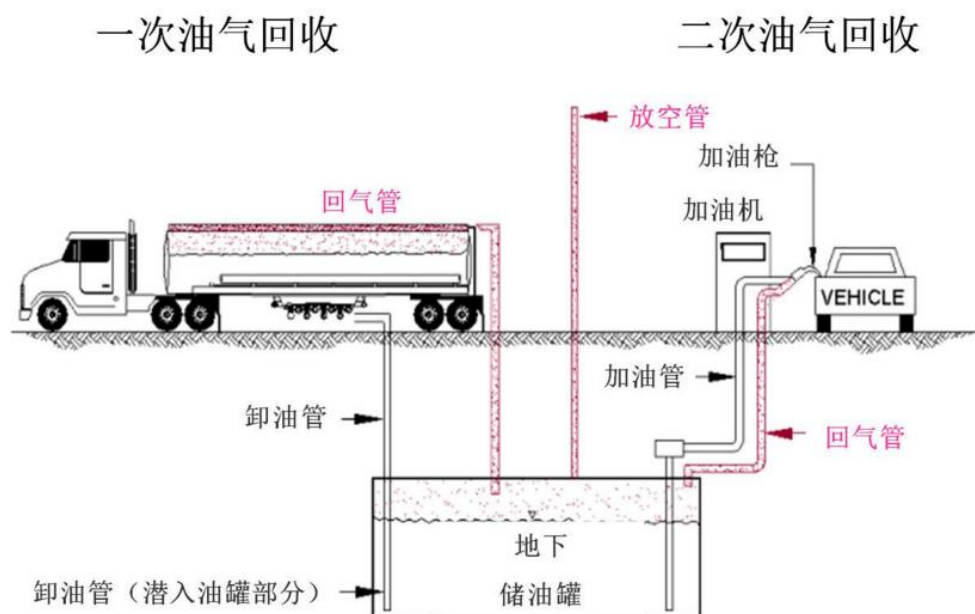
图 6 加油站油气回收装置工艺流程图
