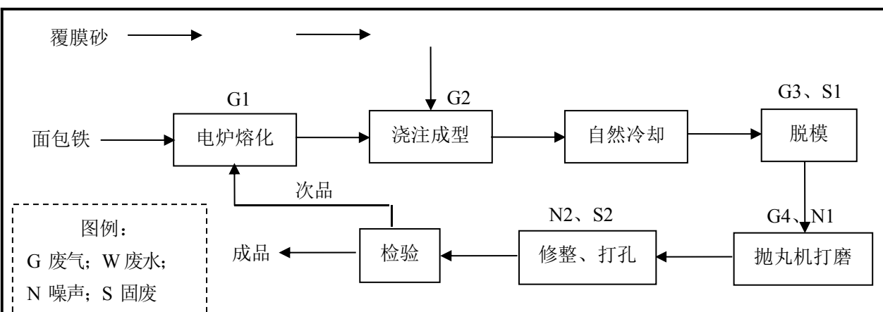
图 2 现有工程生产工艺流程及排污节点
