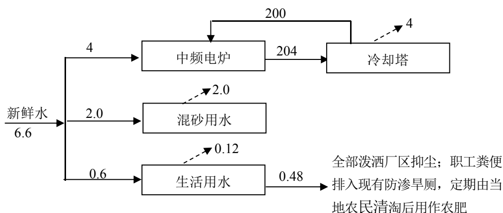
图 1 技改工程水平衡图 单位 m 3 /d
