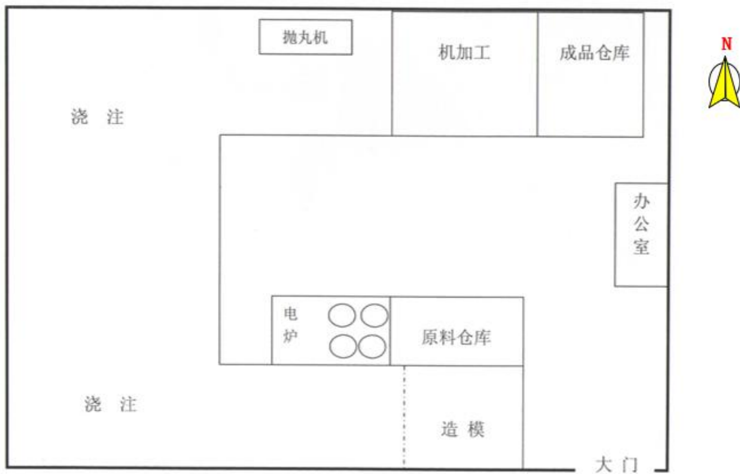
附图 4 技改前原厂 区平面布置图
