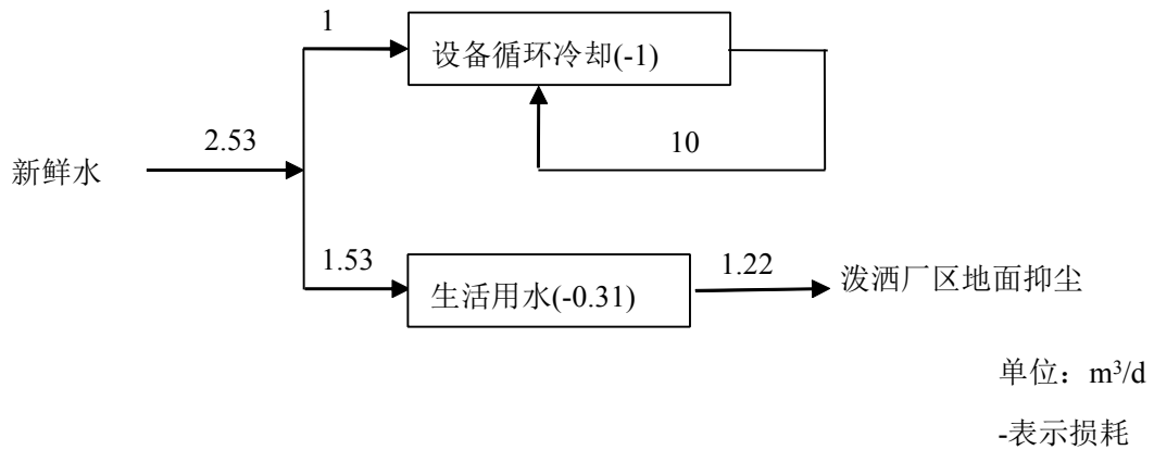
图 1 建设项目水量平衡图
