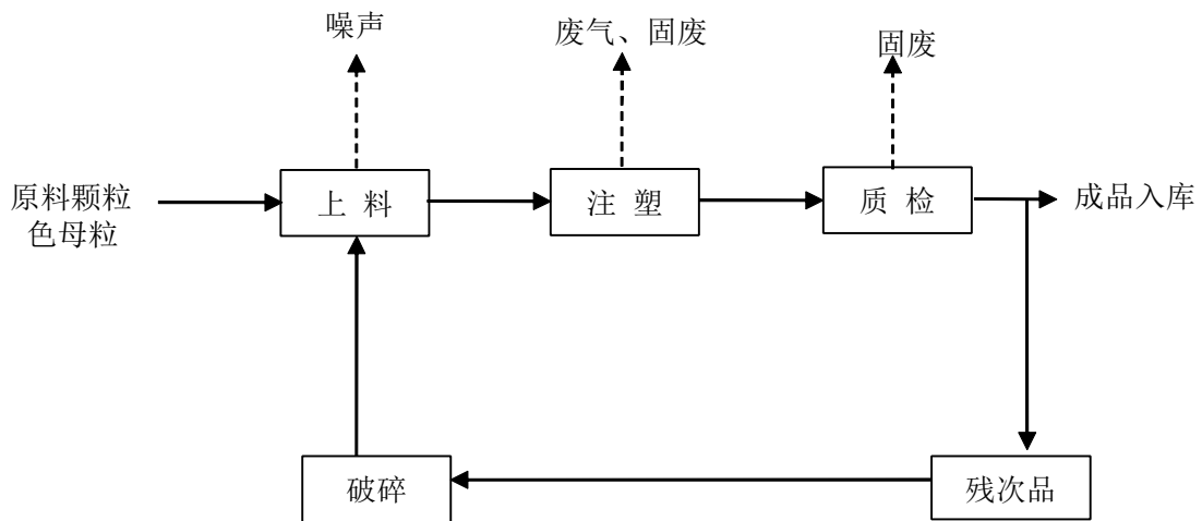
图2 项目工艺流程图
