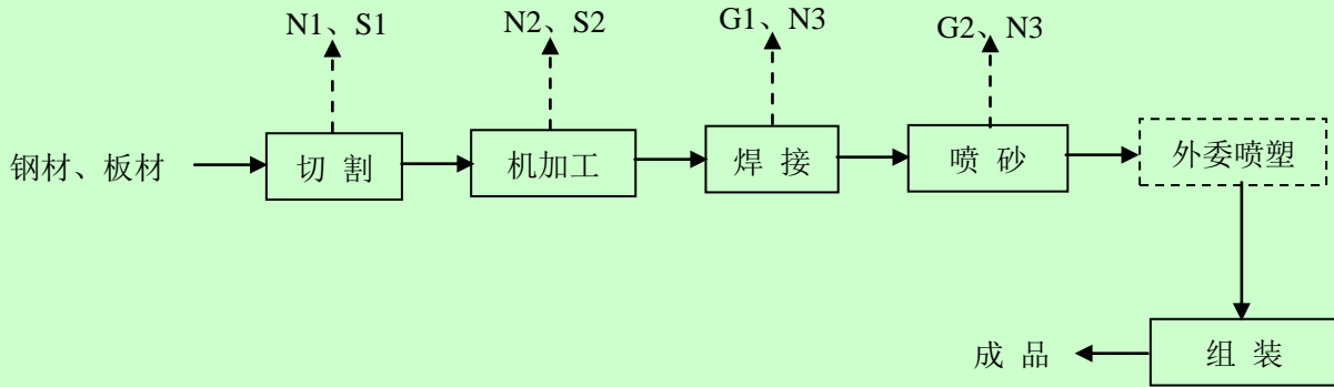
图2 钢质文教体育用品生产工艺流程图
