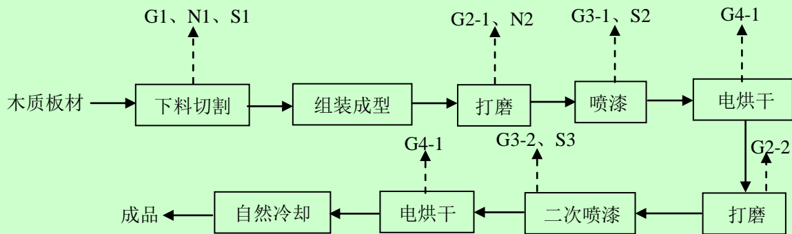
图3 木质文教体育用品生产工艺流程图
