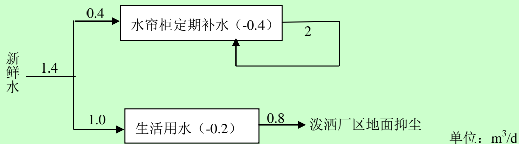
图 1 全厂水量平衡图
