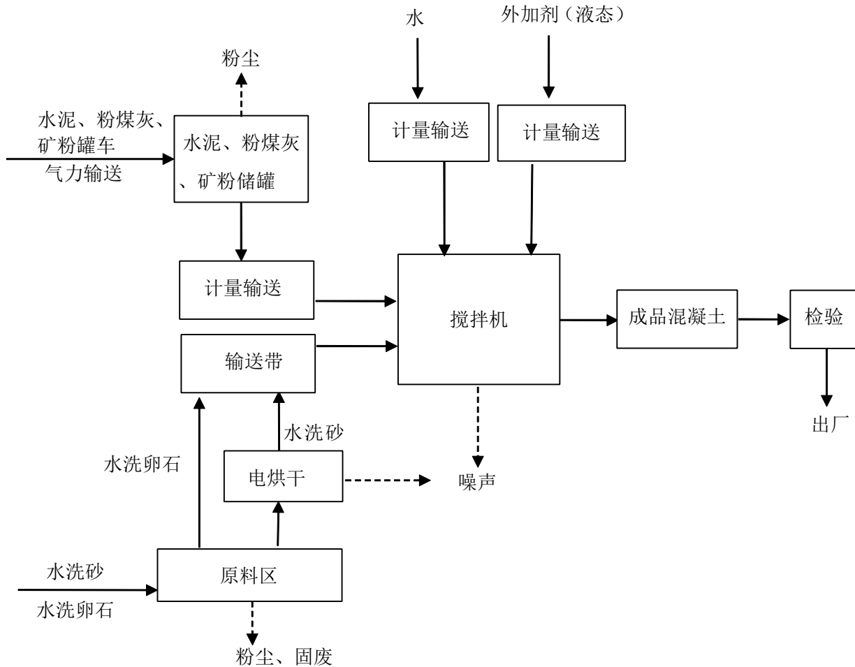
图 2 生产工艺流程图
