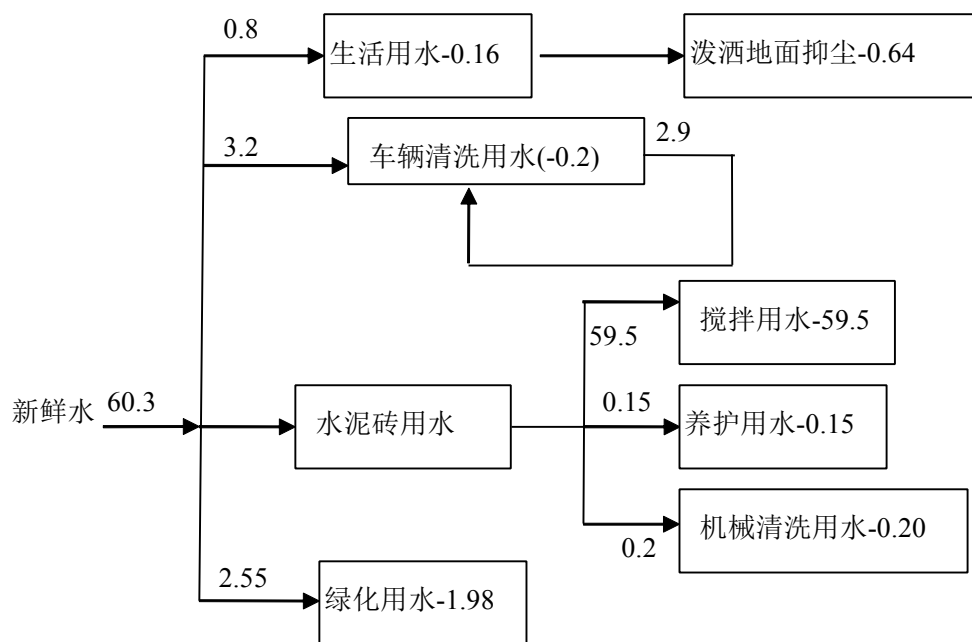
图 1 建设项目水量平衡图
