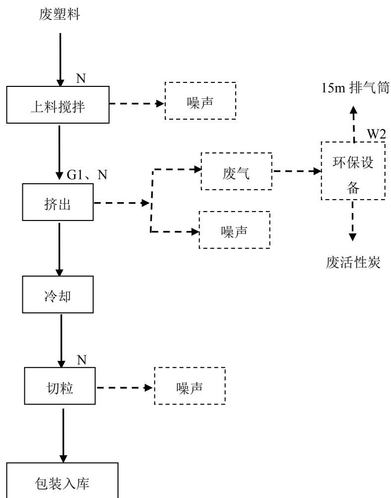
图 2 生产工艺流程及污节点排图
