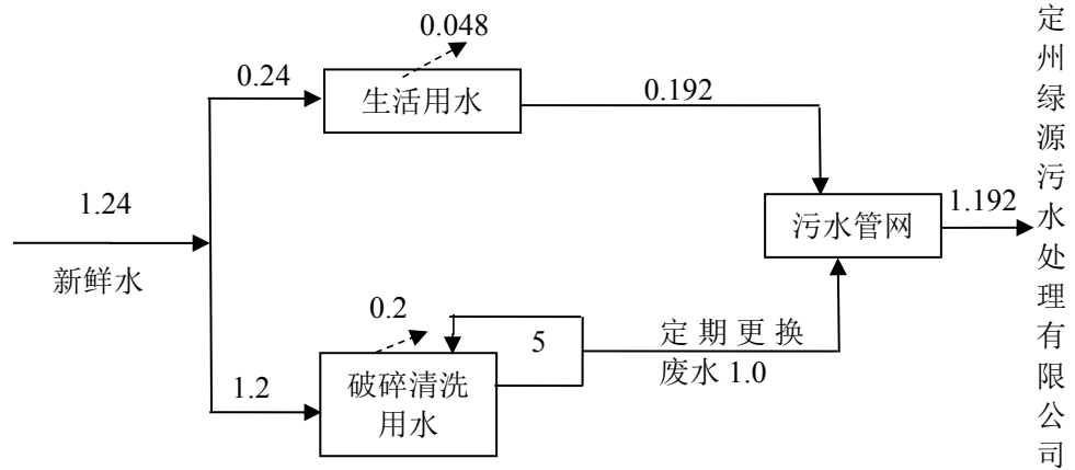
图 1 项目水量平衡图 单位：m 3 /d
