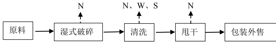
图 2 工艺流程及排污节点图
