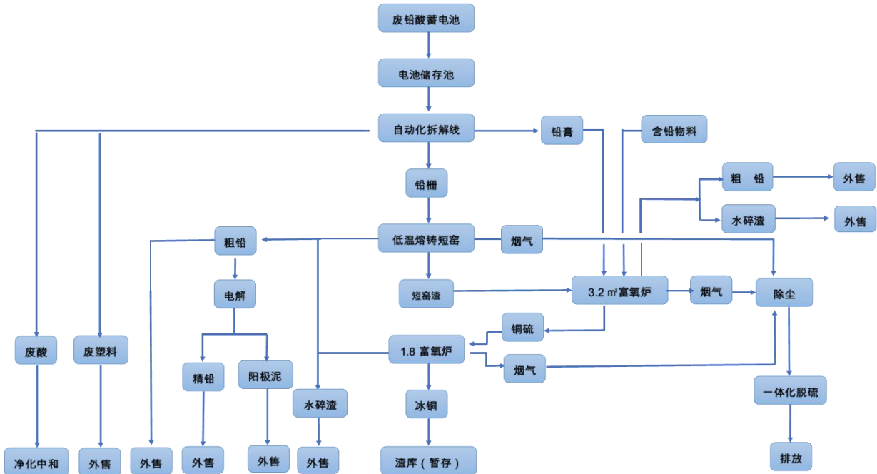
废铅酸蓄电池及含铅物料处置总工艺流程图
